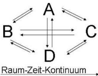
Quantenphysikalisches Denkmodell (Hecht und Hecht-Savoley, 2008)
